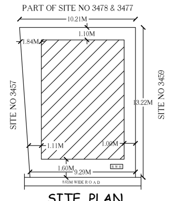
SITE PLAN 1:200
