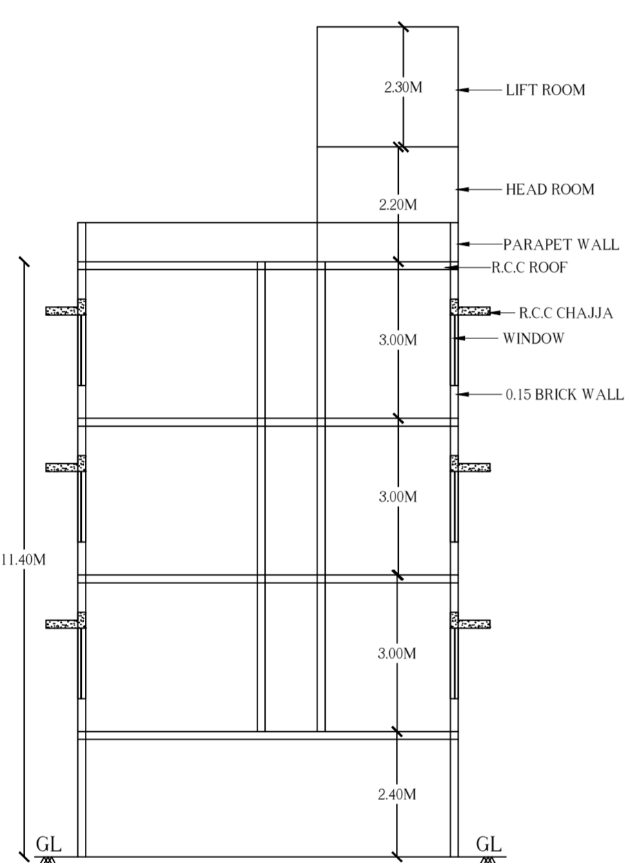
SECTION A-A
